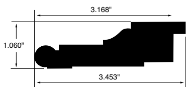
CASING WSCA2A 3.453"x1.060"
