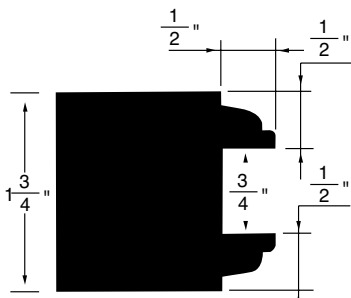
EXTERIOR DOOR WSED1 1/2"x1-3/4"
