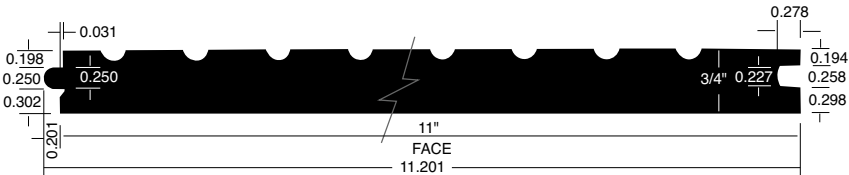
STANDARD SQUARE EDGE T&G BACK RELIEF
